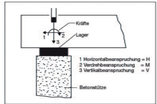
Bild 1 Einwirkende Kräfte
